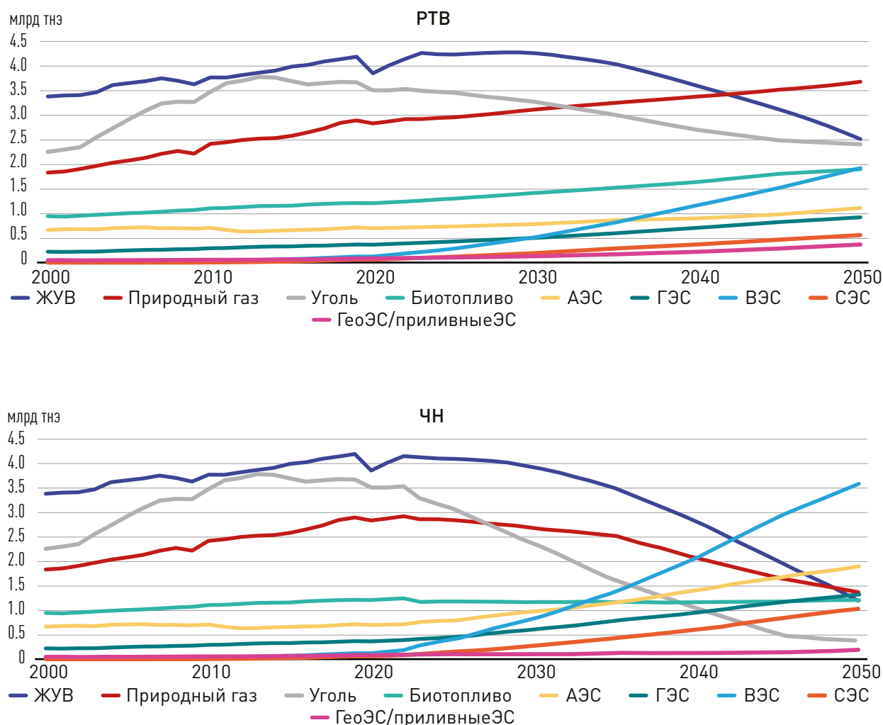
Рис. 10. Динамика потребления первичных ТЭР в 2000–2050 гг.
