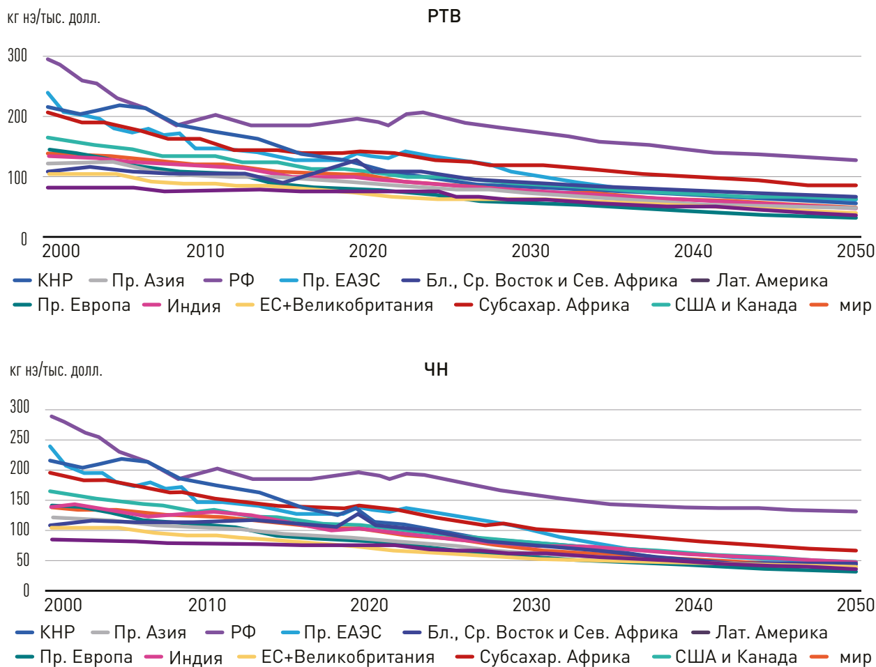
Рис. 7. Динамика энергоёмкости ВВП в макрорегионах и мире в целом
