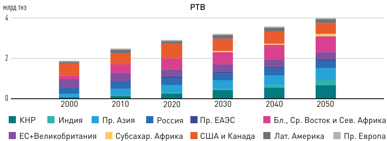
Рис. 29. Региональная структура потребления газа
